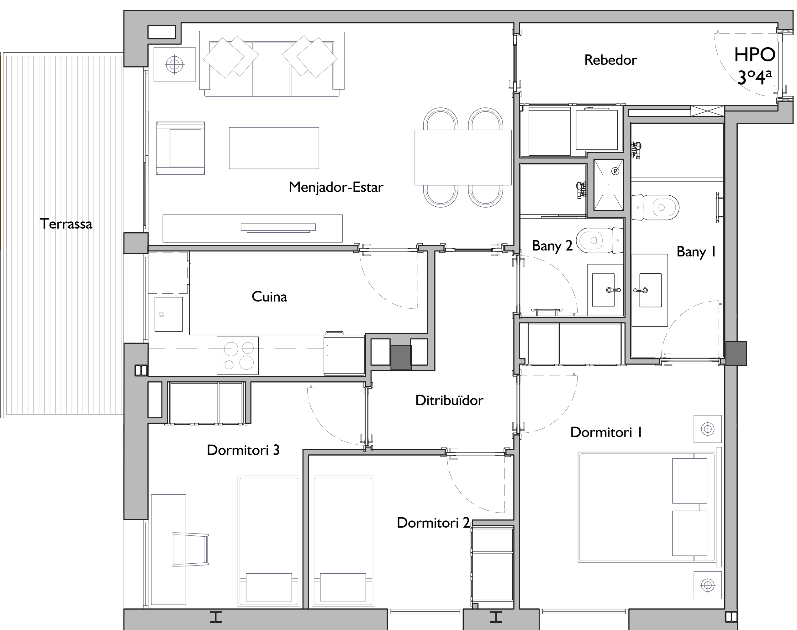
PLANTA 3R 4T
