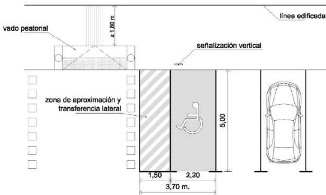
Figura 2. Plaça de aparcament reservada amb accés des de pas de peatons
