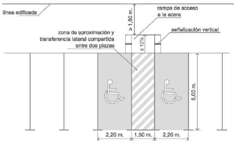
Figura 1. Places de aparcament reservades disposades en perpendicular a la acera i amb accés compartit
