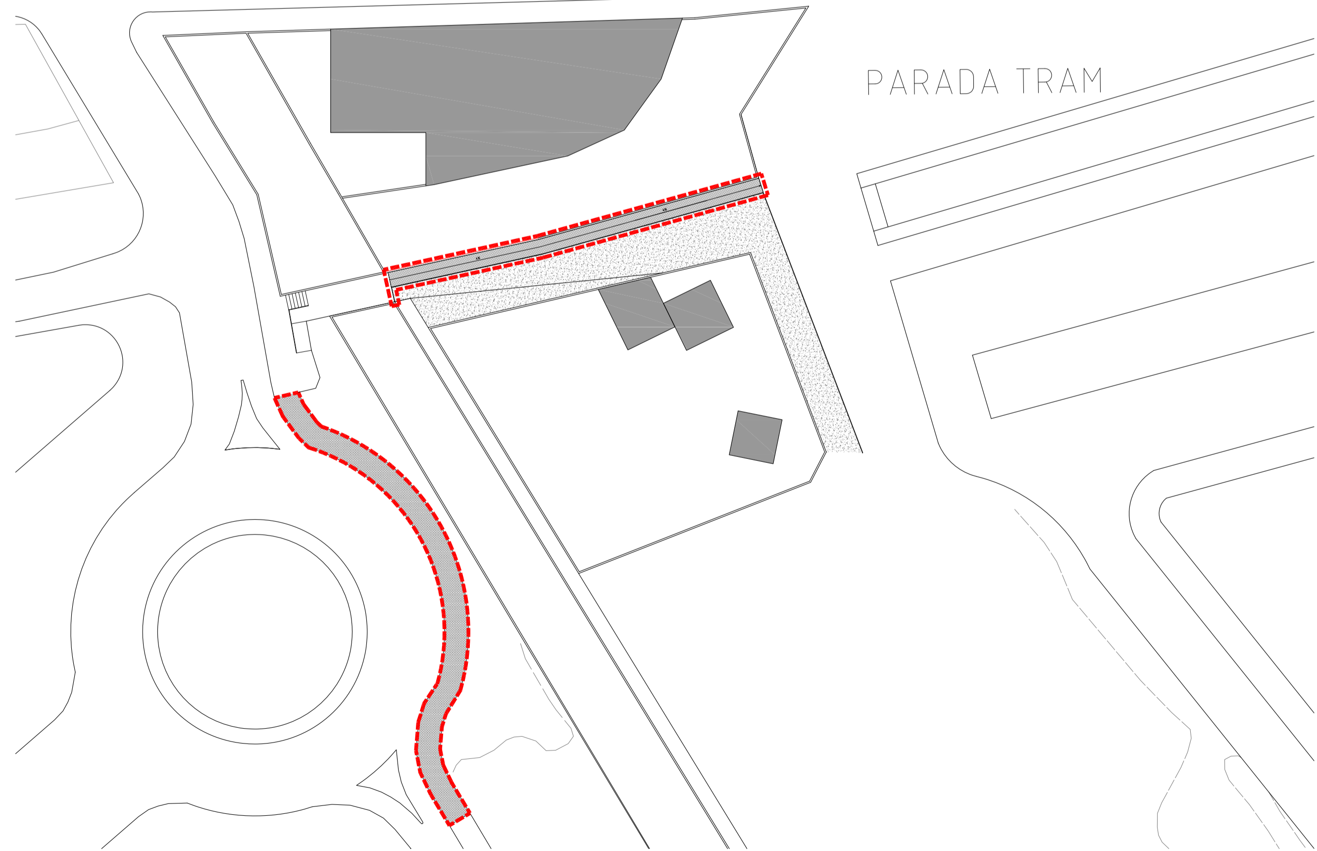
PLANTA PAVIMENTACIÓ I ADAPTACIÓ ACCÉS AL TRAM DE SANT FELIU (IMATGE 2)
