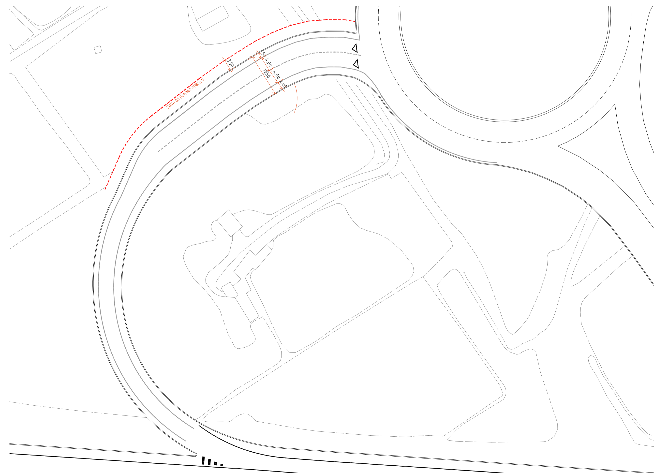
DESDOBLAMENT ULTIM TRAM CARRIL DESACELERACIÓ B-23. e.1/500
