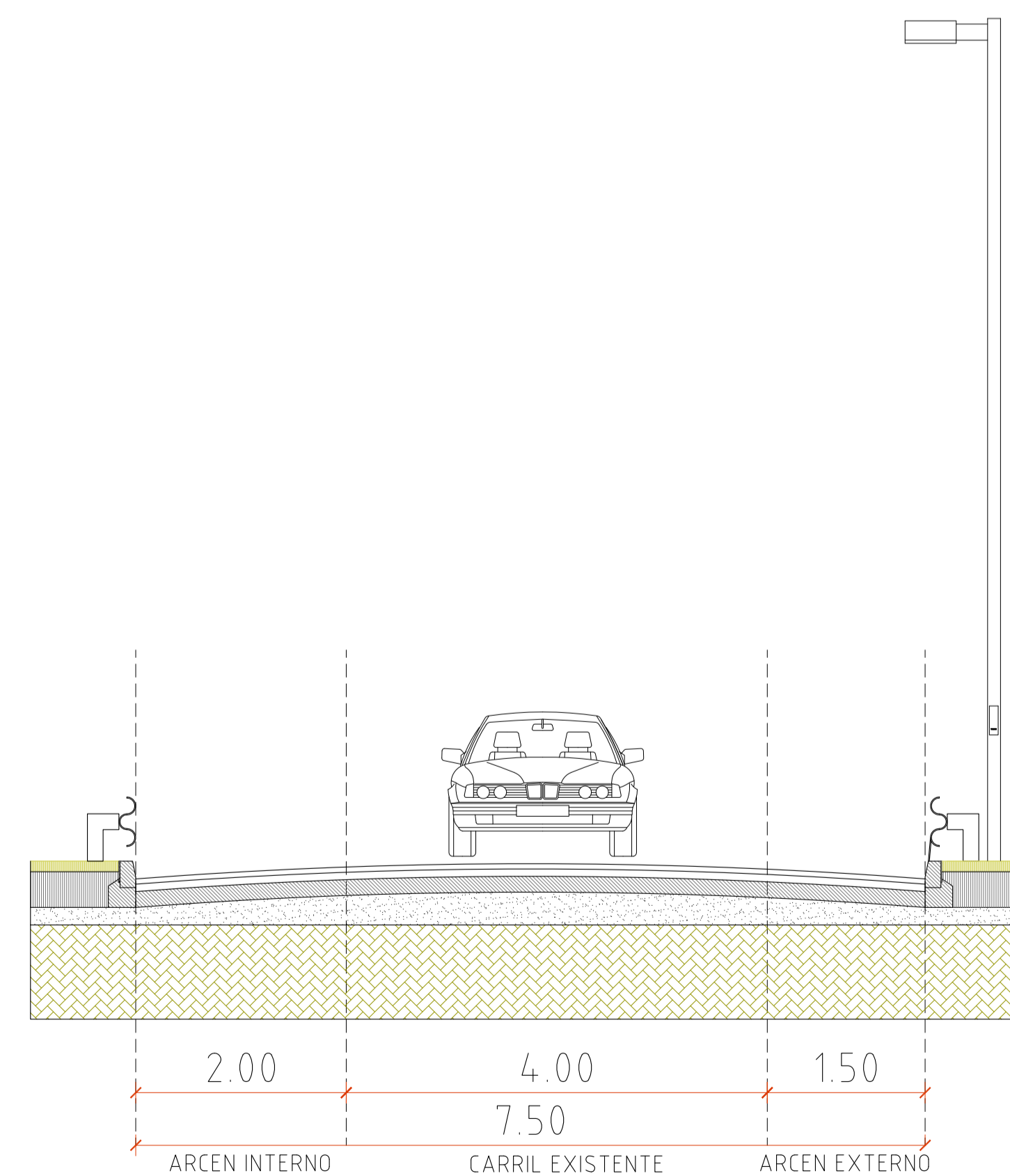
SECCIÓ CARRIL DESACELERACIÓ B-23 EXISTENTE
