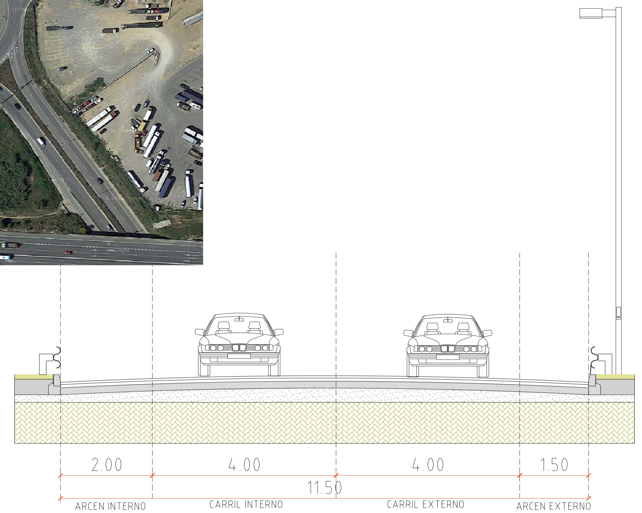
SECCIÓ CARRIL DESACELERACIÓ B-23 - PROPUESTA
