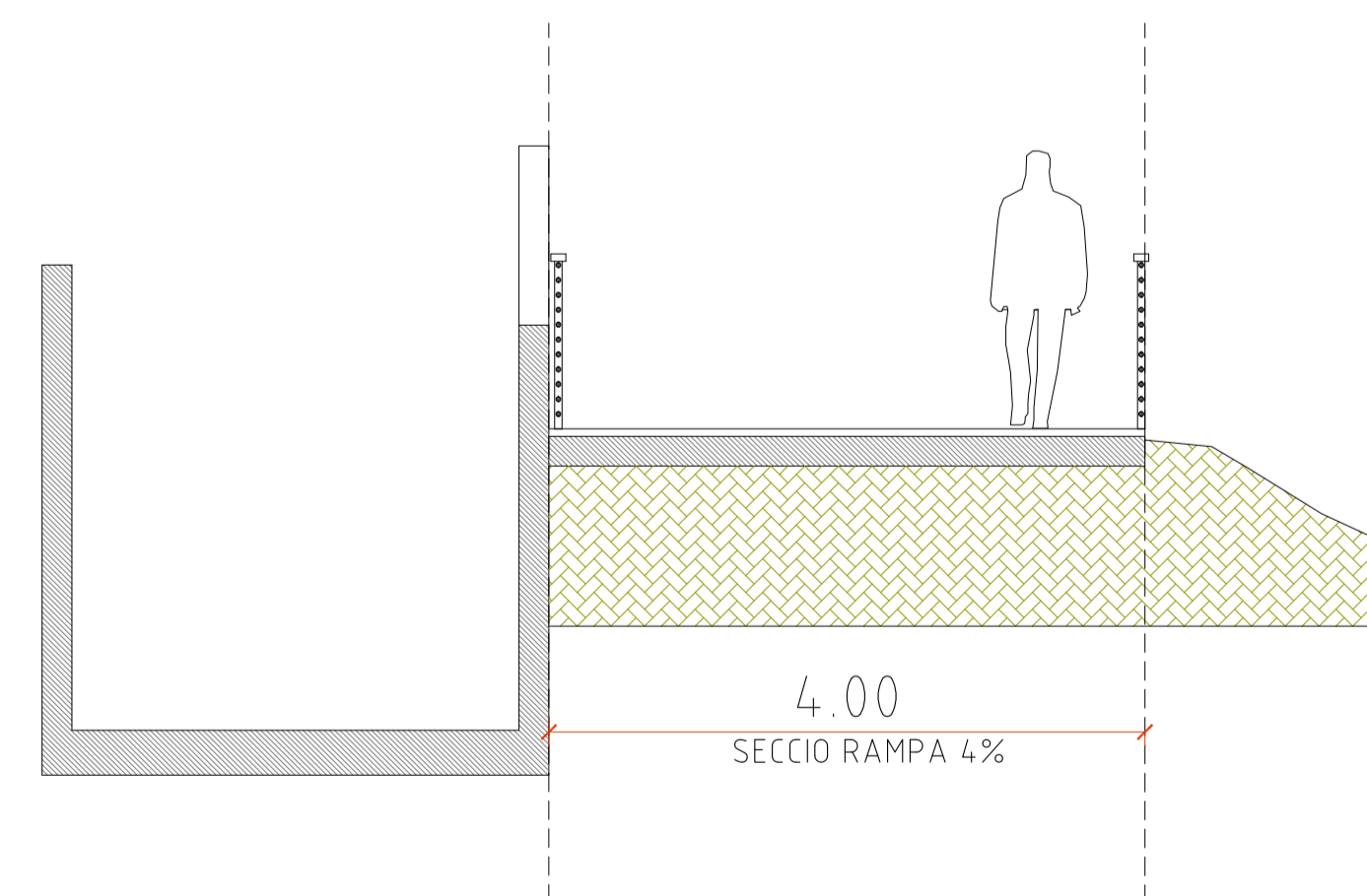
SECCIÓ RAMPA ACCÈS AL TRAM e: 1/50
