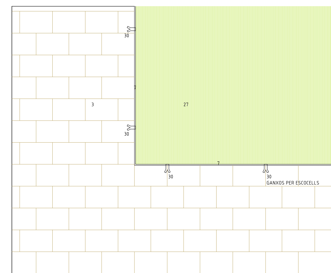
DETALL PAVIMENT DE LLOSES CANIGÓ AMB ZONES DE GESPA
