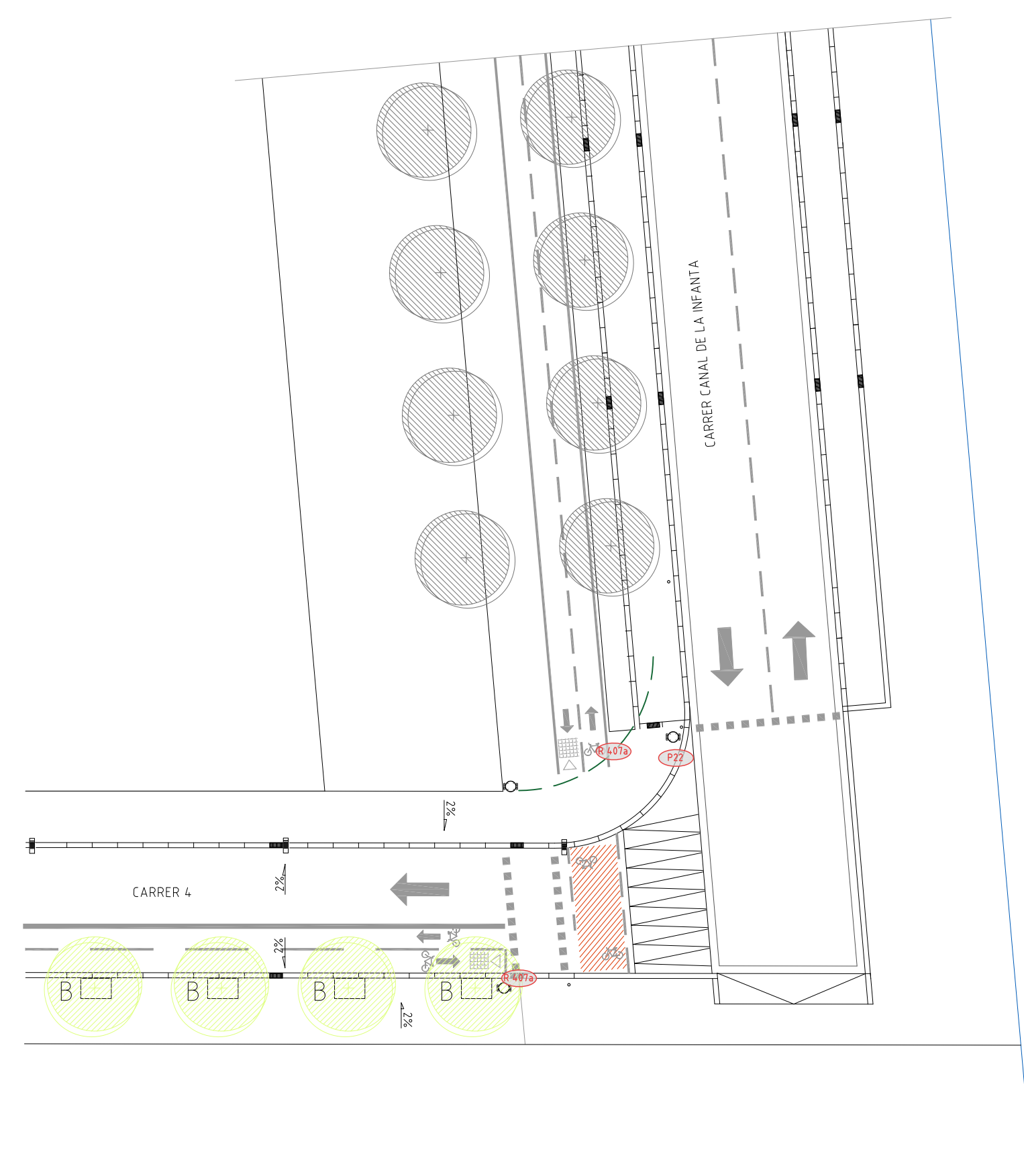
ENCREUAMENT VIAL 4 AMB EXISTENT CARRER CANAL DE LA INFANTA
