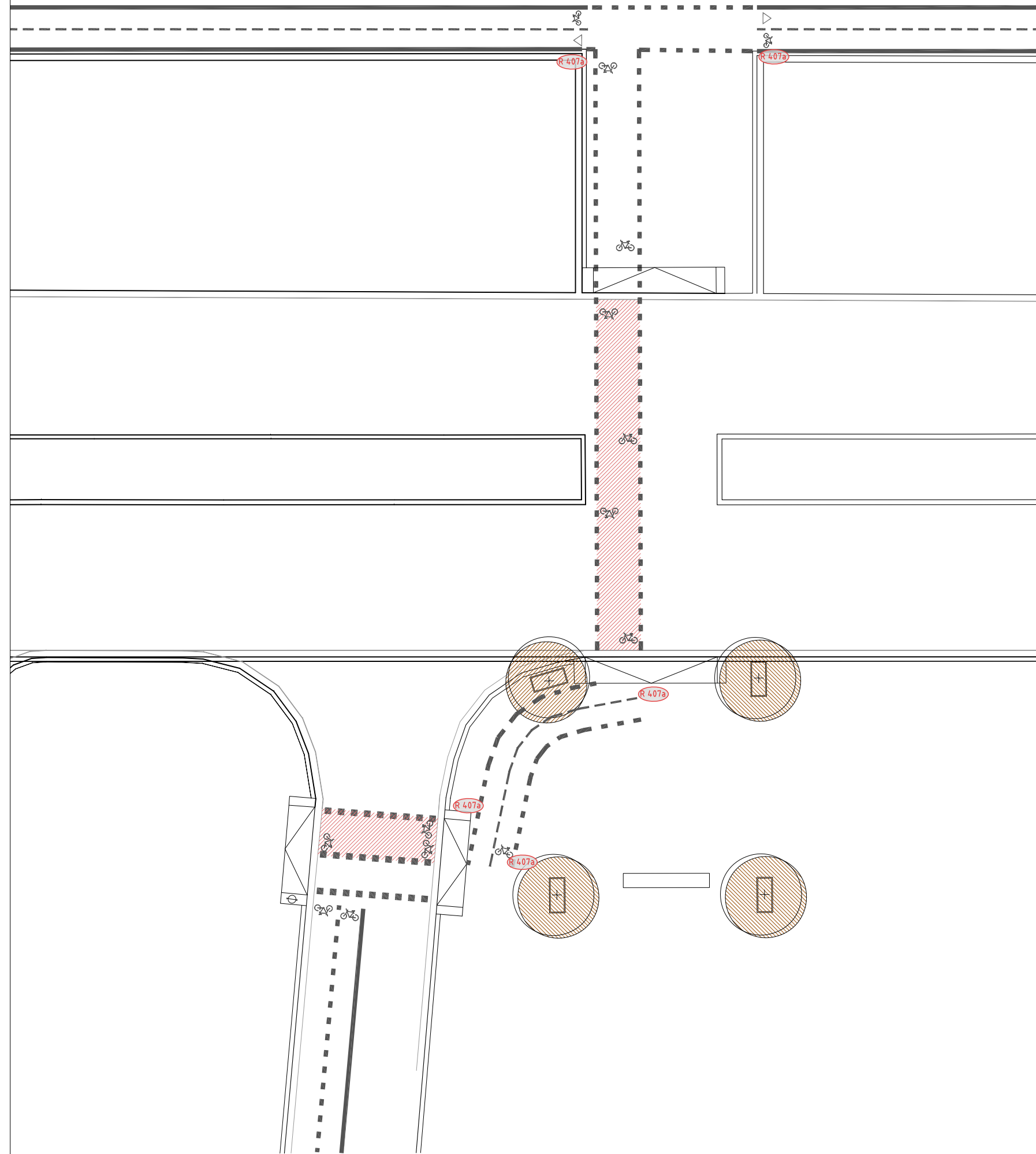
UNIÓ CARRIL BICI EXISTENT AV. 11 DE SETEMBRE AMB CARRIL BICI NOVA CREACIÓ CARRER DEL MIG
