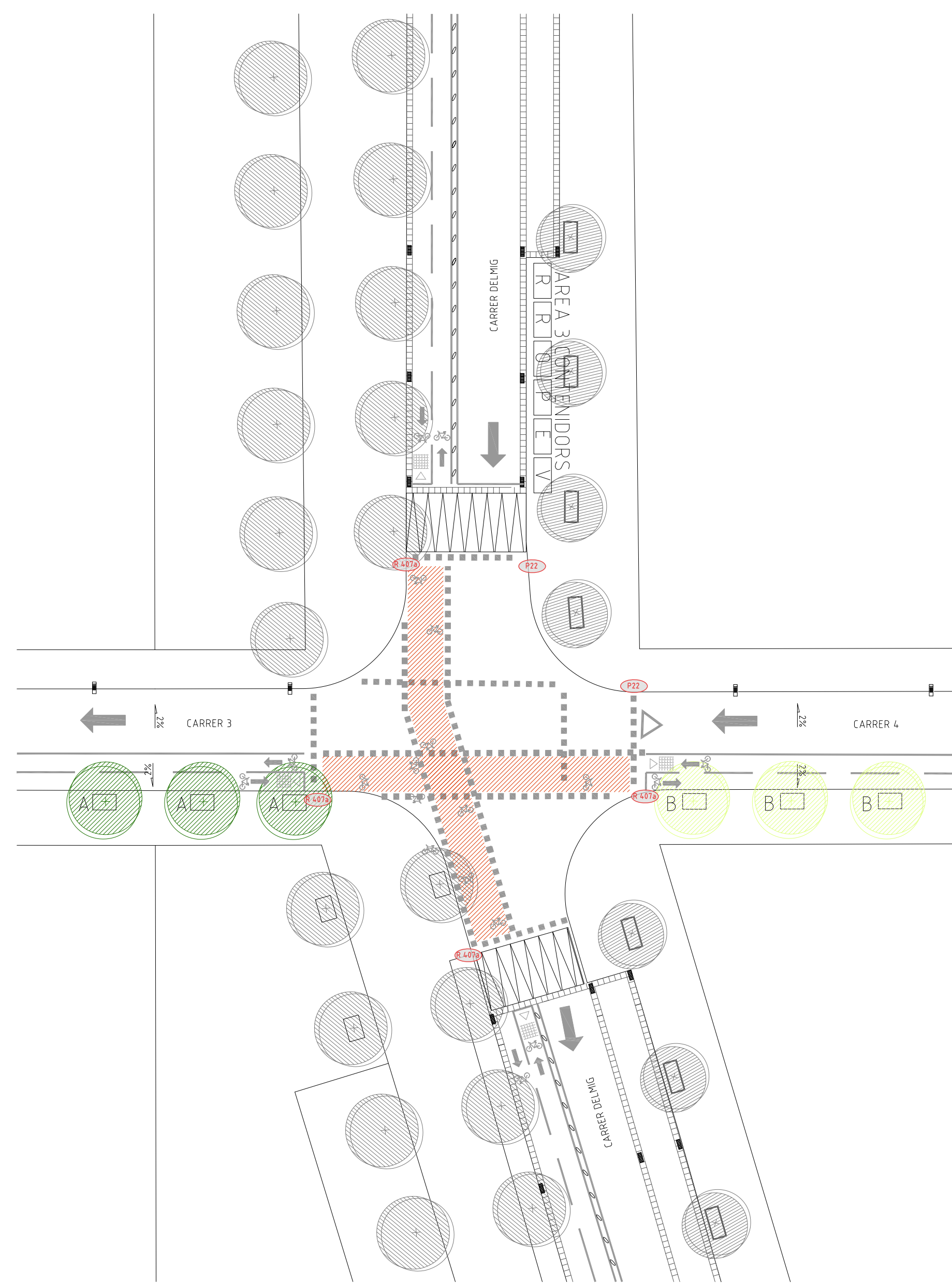
ENCREUAMENT VIALS 3 I 4 AMB CARRER DEL MIG
